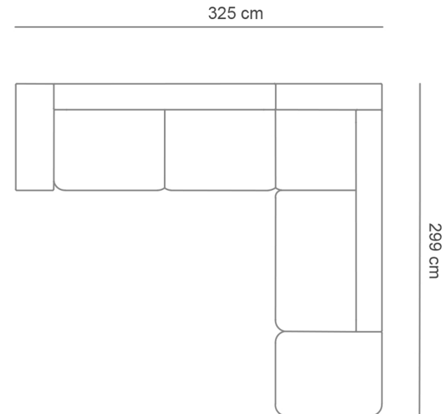
EXEMPLU COLTAR CU 2 CANAPELE DE 190 cm + POUF
